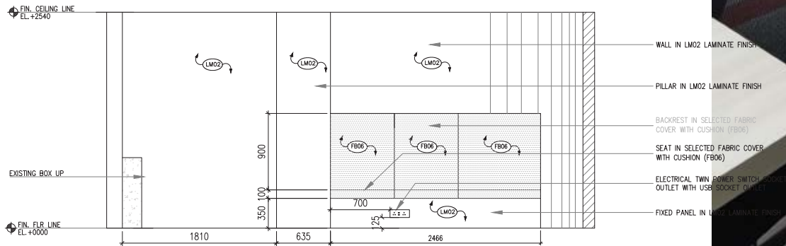
ELE ELEVATION J02 SCALE 1 : 40
