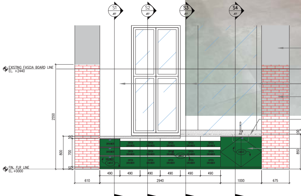
ELE ELEVATION J07 SCALE 1 : 40
