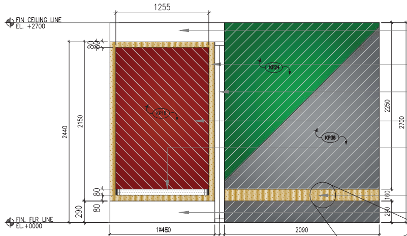
ELE ELEVATION J10 SCALE 1 : 40
