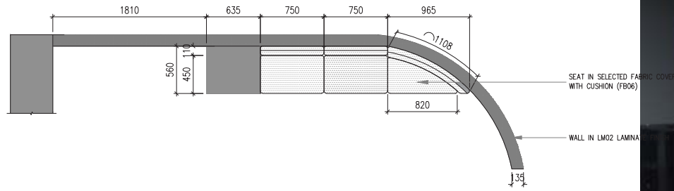
KP KEY PLAN J02 SCALE 1 : 40
