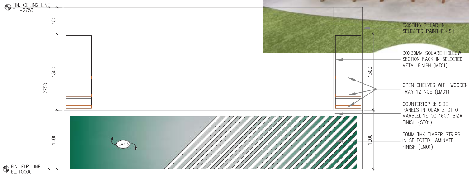
ELE J06 | ELEVATION A SCALE 1 : 40
