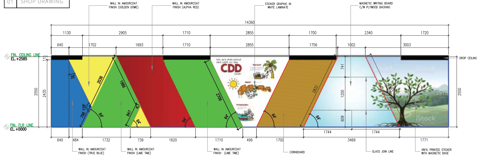
ELE FRONT ELEVATION J13 SCALE 1 : 50
