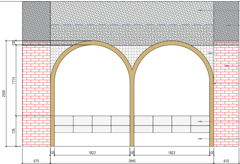
ELE ELEVATION J08 SCALE 1:30
