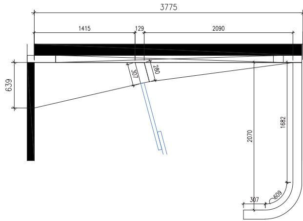
KP KEY PLAN J10 SCALE 1 : 40
